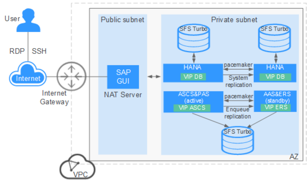
图 2-8 推荐的 SAP NetWeaver 分布式 HA 部署
